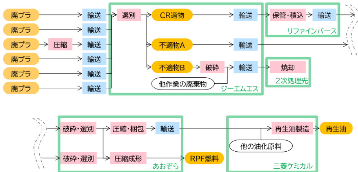
図10 本事業にて試行した処理フロー・物質フロー
