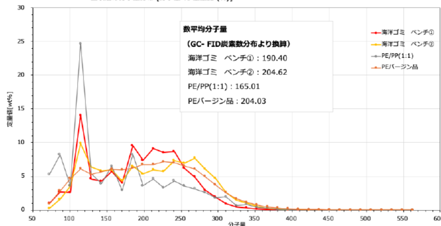
回収油の分子量分布 [分子量 vs 重量比 (%)]
