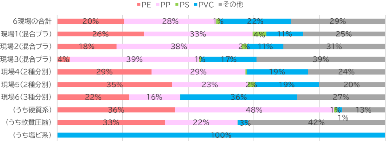
図12 本実証の物質収支とステージ区分別の発生割合（重量比）
