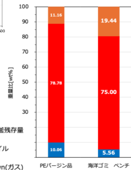
マテリアルバランス (重量比)
