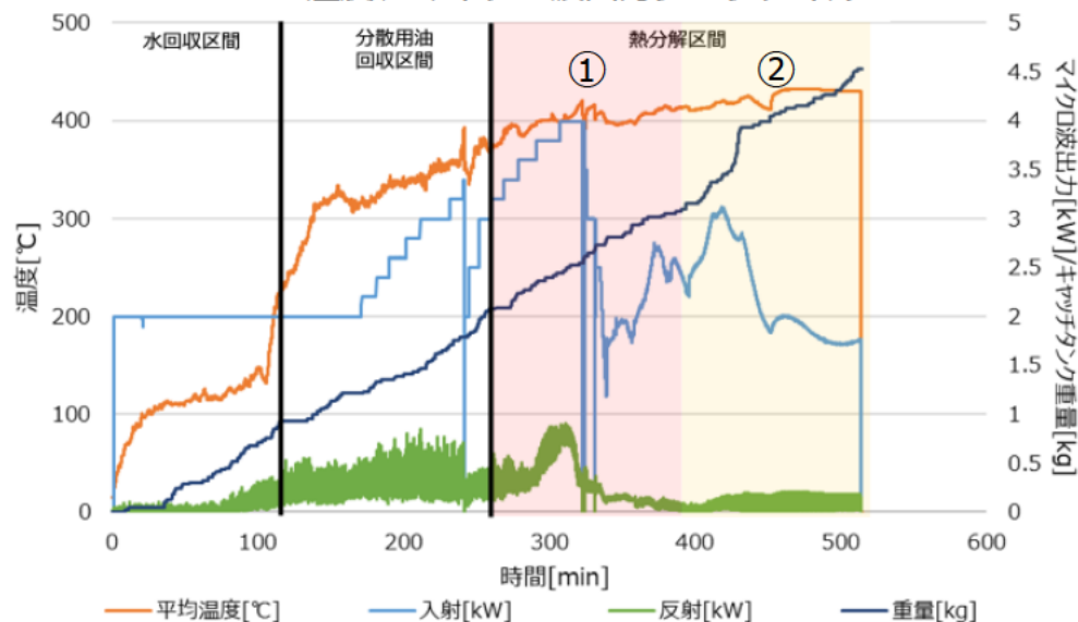
温度、マイクロ波出力プロファイル
