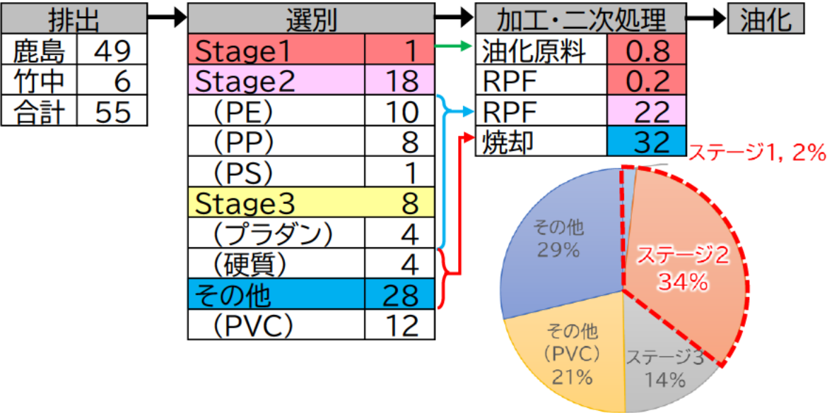
図11 本実証の物質収支とステージ区分別の発生割合（単位：トン）
