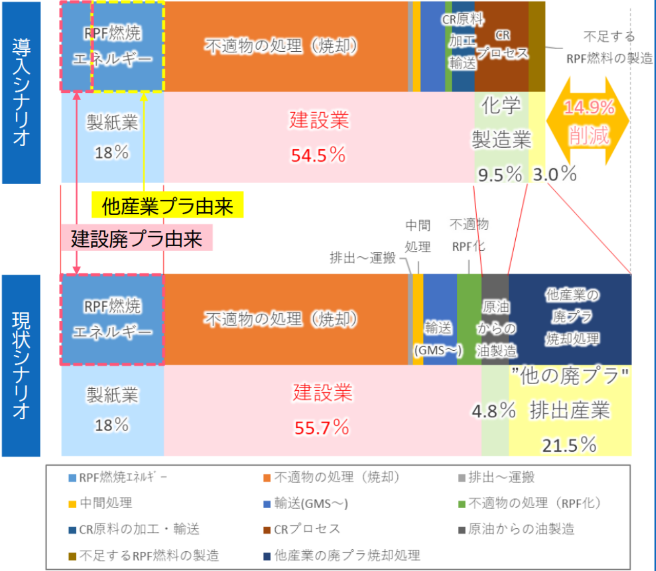
図14 現状シナリオ・導入シナリオのCO2排出量の算出結果
